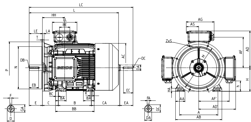
IM B35 安装结构方式 Type of construction IM B35
