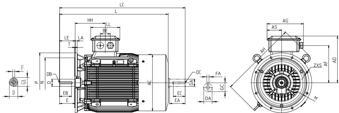
IM B35 安装结构方式 Type of construction IM B35
